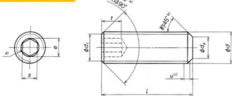
六角穴付き止めねじ
